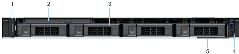
Ilustración 2. Vista frontal de un sistema de 4 unidades de 3,5 pulgadas
