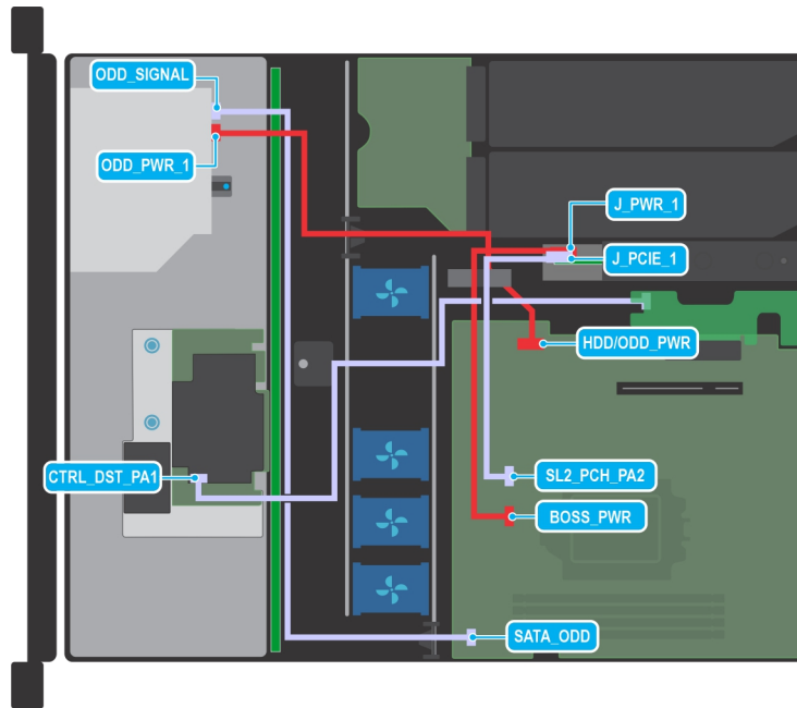
Ilustración 25. Enrutamiento de cables: backplane de 4 unidades SAS o SATA de 3,5 in con fPERC y tarjeta Boot Optimized Storage Subsystem
