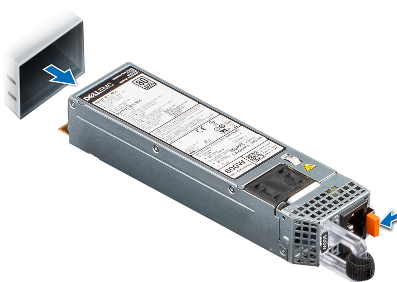
Ilustración 67. Extracción de una fuente de alimentación
