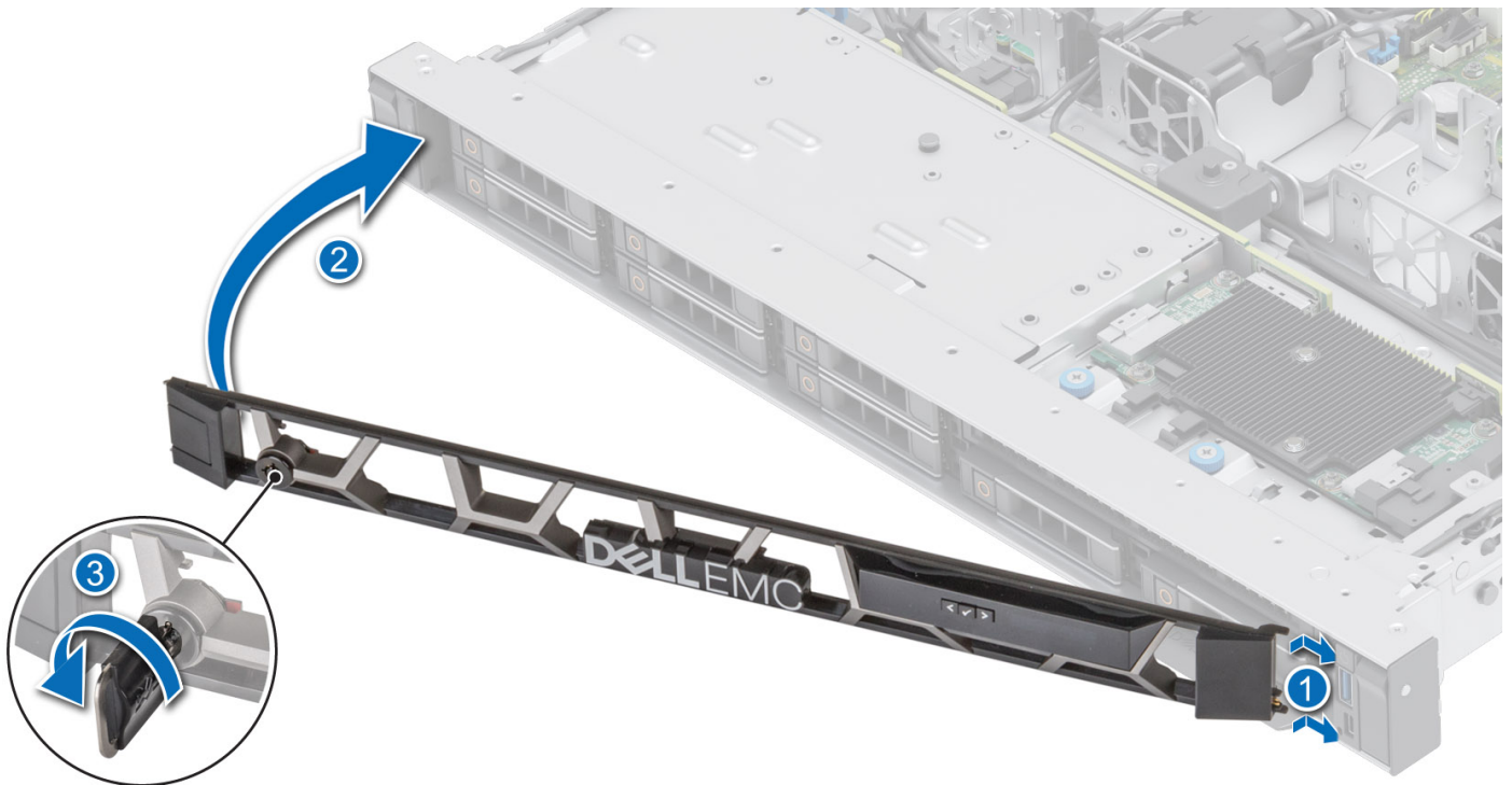
Ilustración 10. Instalación del bisel frontal con el panel LCD
